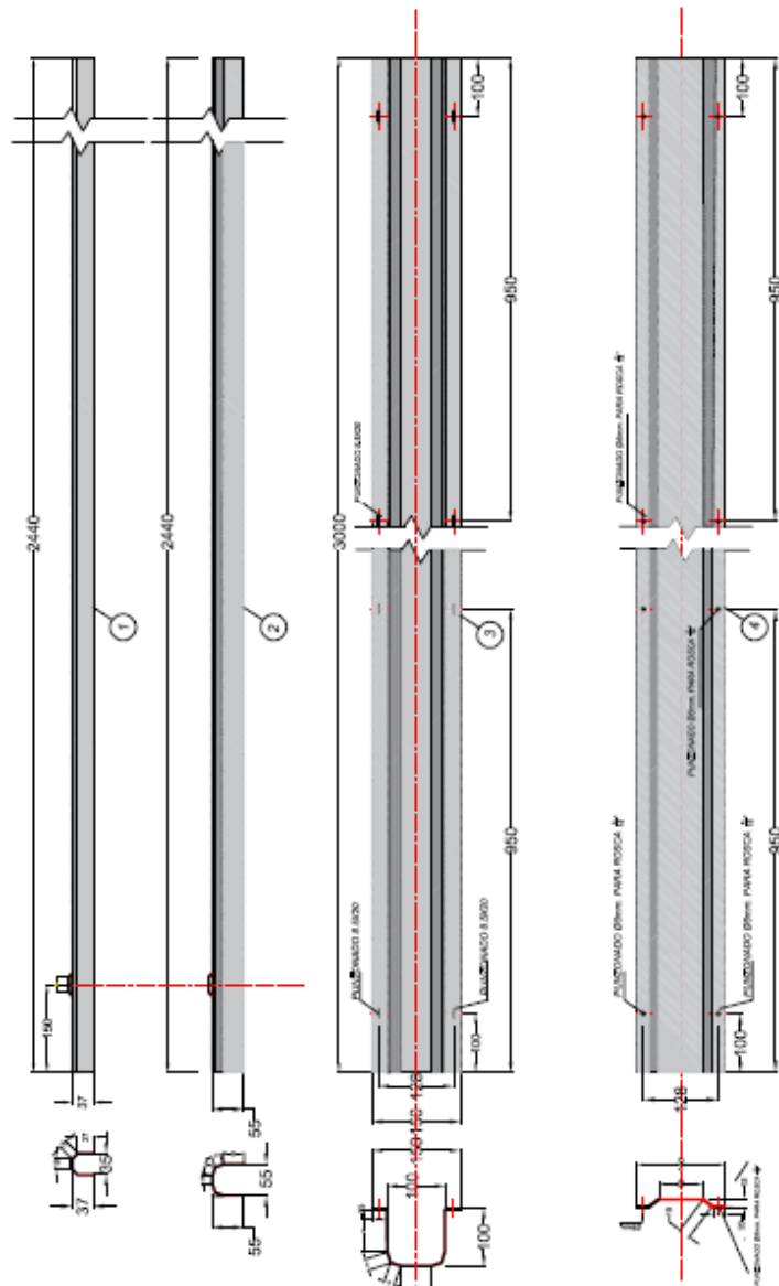
PIEZA Nº 4 CHAPA PLEGADA CON PUNZONADO ESP. 3mm x 3m. Cod. 751115
